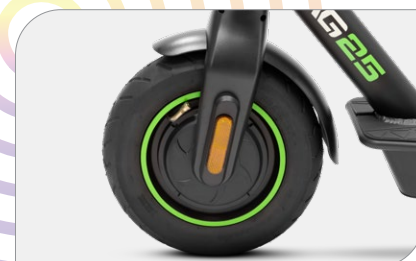
Motore brushless 350 W, 17 Nm
