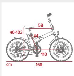
Dimensions du vélo électrique
