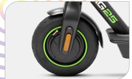
Moteur brushless : 350 W, 17 Nm
