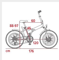
Dimensions du vélo électrique
