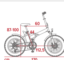
Dimensioni e-bike
