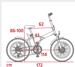
Dimensions du vélo électrique
