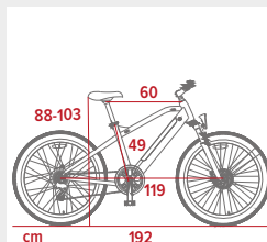
Dimensions du vélo électrique
