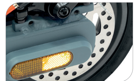
Sistema frenante con tecnologia KERS integrata
